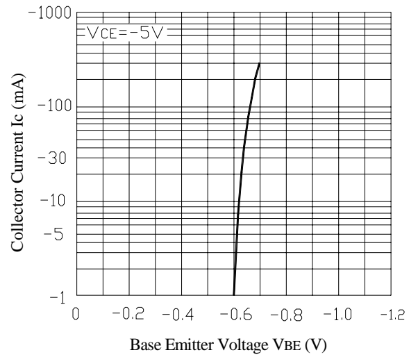
I_C - V_{BE}
